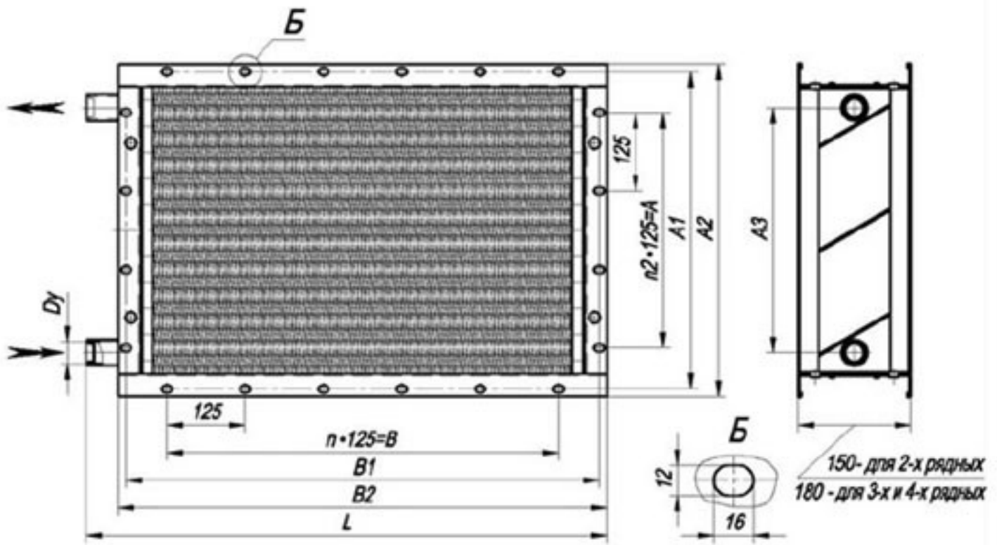
Рис. 1. Калорифер КСк 2-10 размеры, мм
