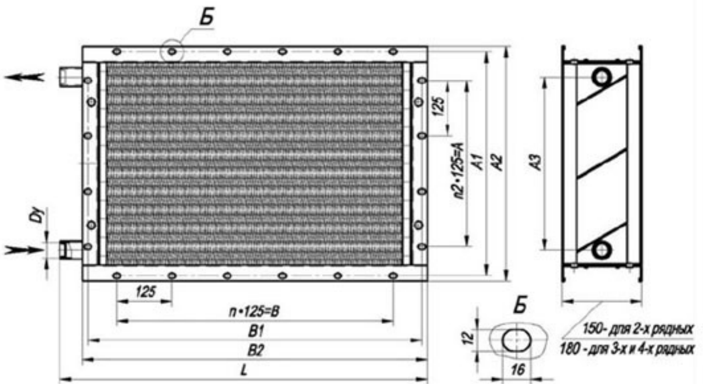
Рис. 1. Калорифер КСк 4-9 размеры, мм
