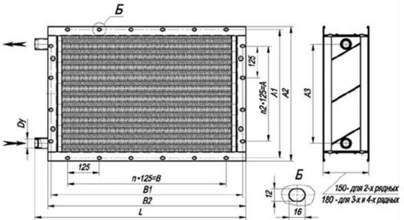
Рис. 1. Калорифер КСк 2-2. Размеры, мм
